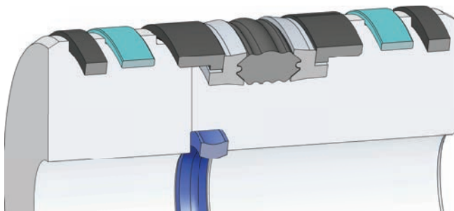
A403 Kapak Keçesi
