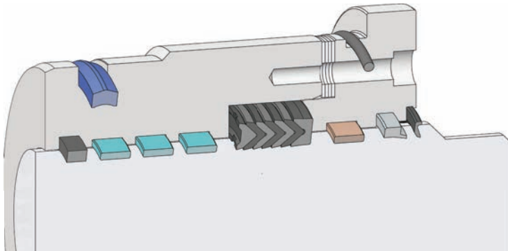
A404 Kapak Keçesi
