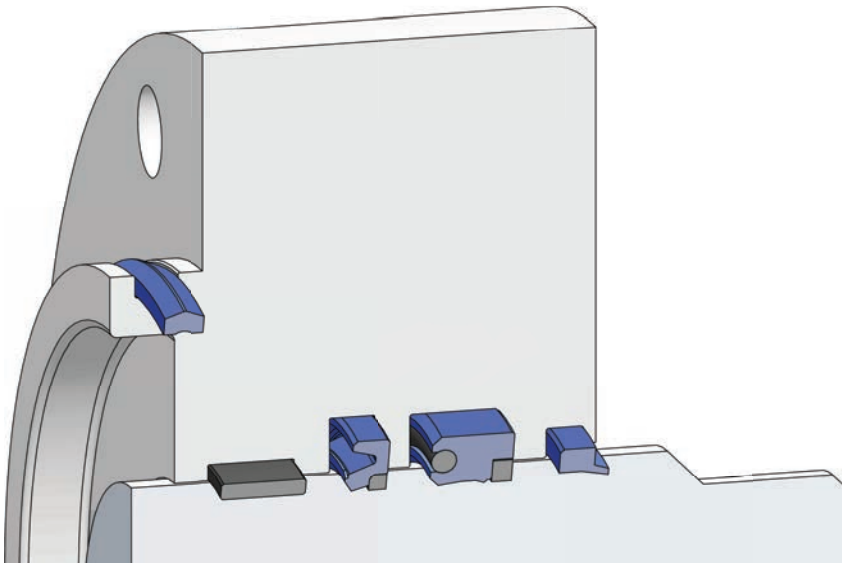
A404 Kapak Keçesi
