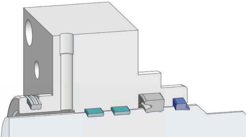
A202 Toz Keçesi
