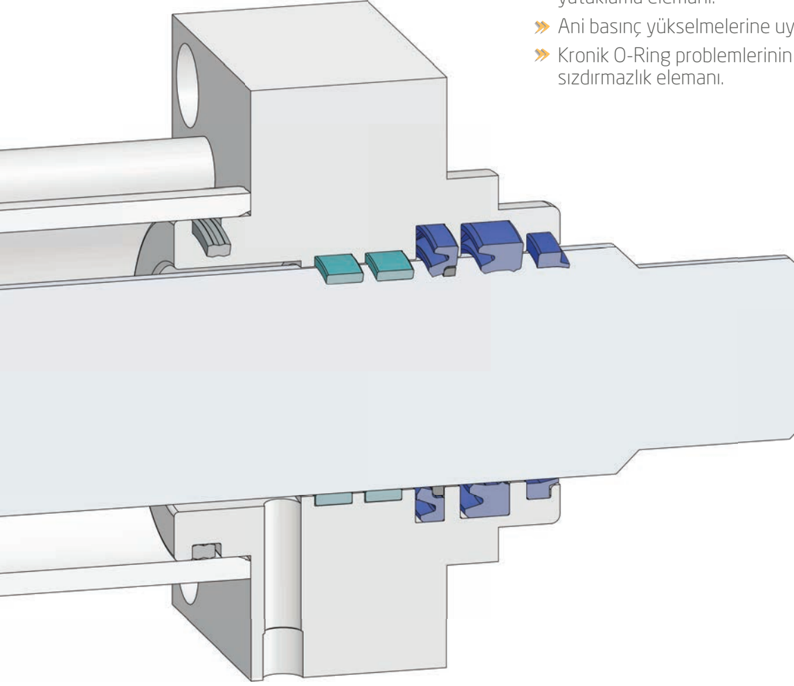
A406 Statik Sızdırmazlık Keçesi
